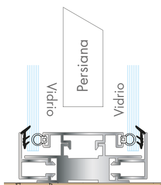
División de oficina doble
